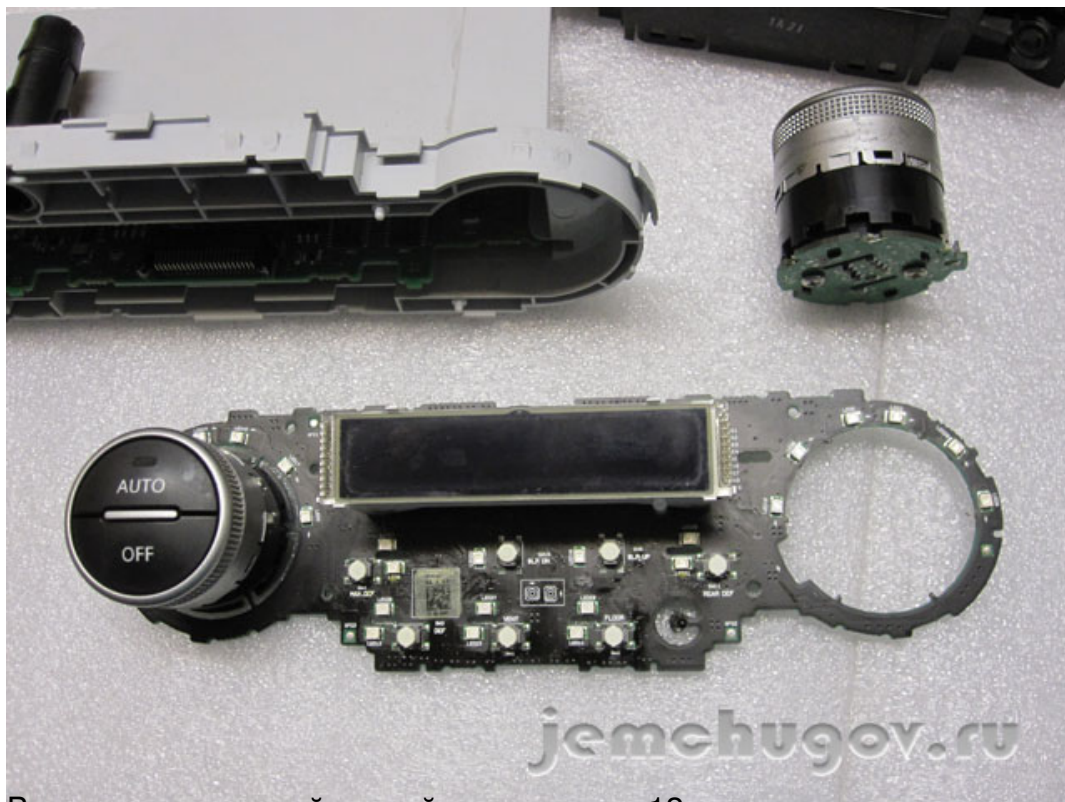
Вместе с оторванной ручкой повреждены 12 дорожек на плате
